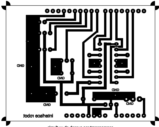
circuit vu de dessus par transparence
